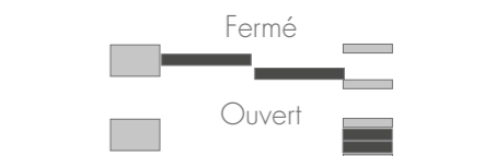
Coulissants à galandage 2 vantaux, 2 rails, ouverture totale (existe aussi en 3 vtx 3 rails et 4 vtx 2 rails)
