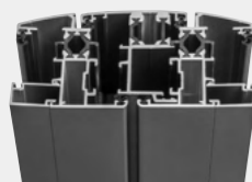
Vue intérieure avec parclose carrée
